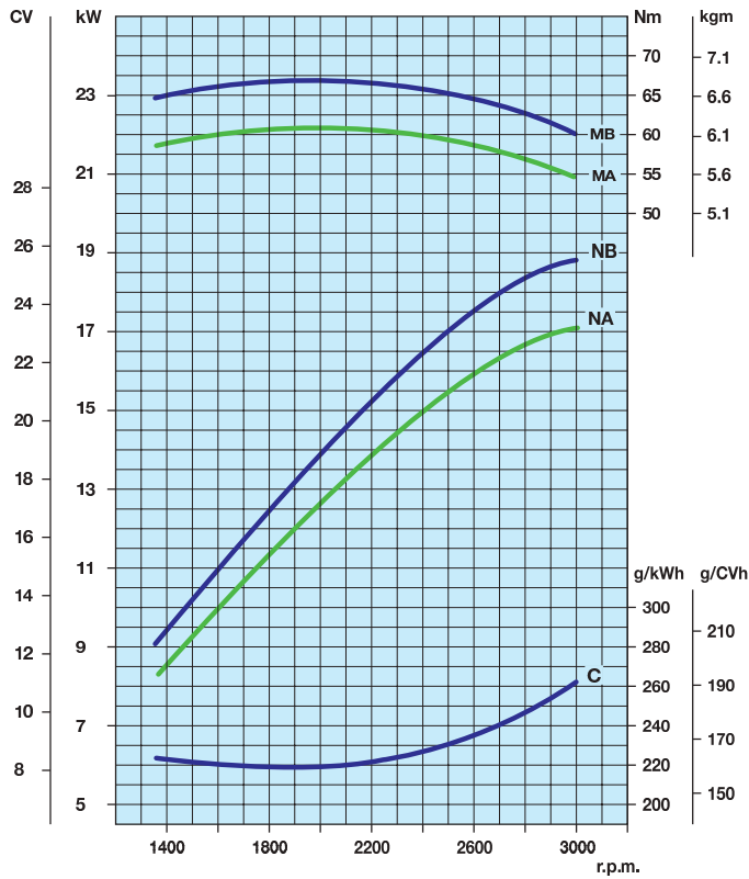
9LD625 @ 3000 giri/min. ■ ● ▲
